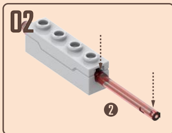
往下轻轻按压②部件尾端，使前端卡扣位置松开
